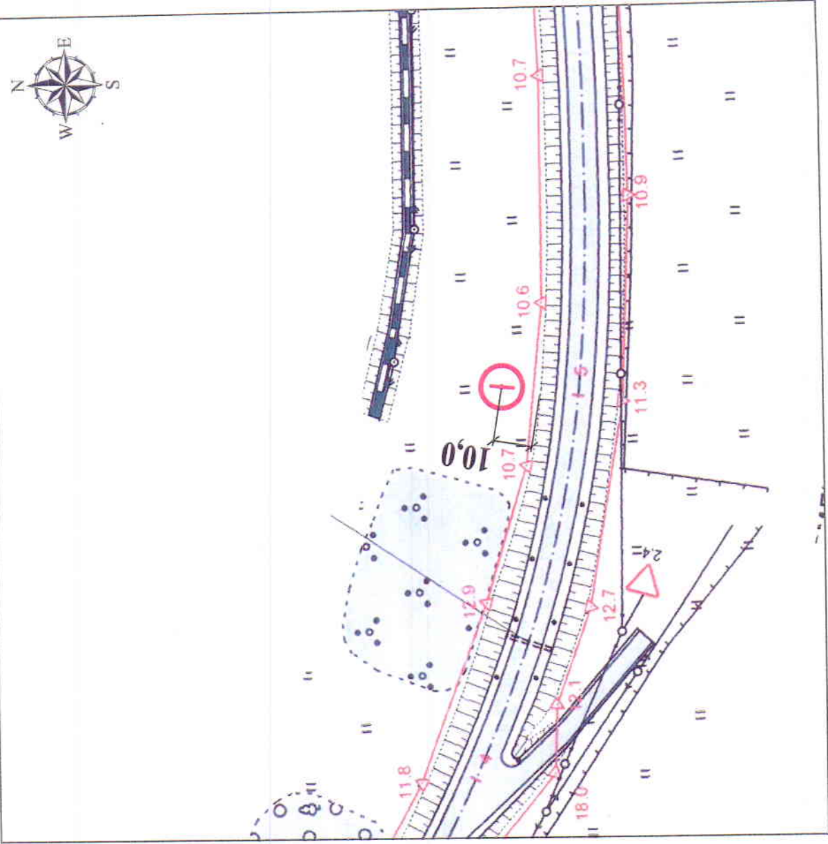
14 км 500 м автомобильной дороги Томск-Аэропорт 69 А-1
